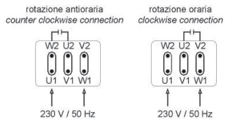
MEC 50/63 regolabile
