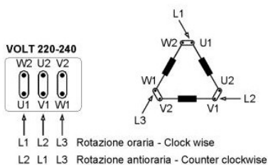
Collegamento a triangolo
