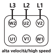
Alta velocità (4/6 poli - 400V/50Hz)
