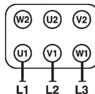
bassa velocità / low speed
