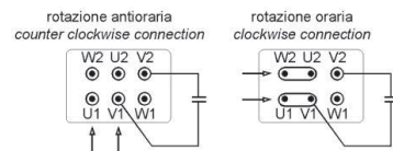
MEC 71/90 regolabile
